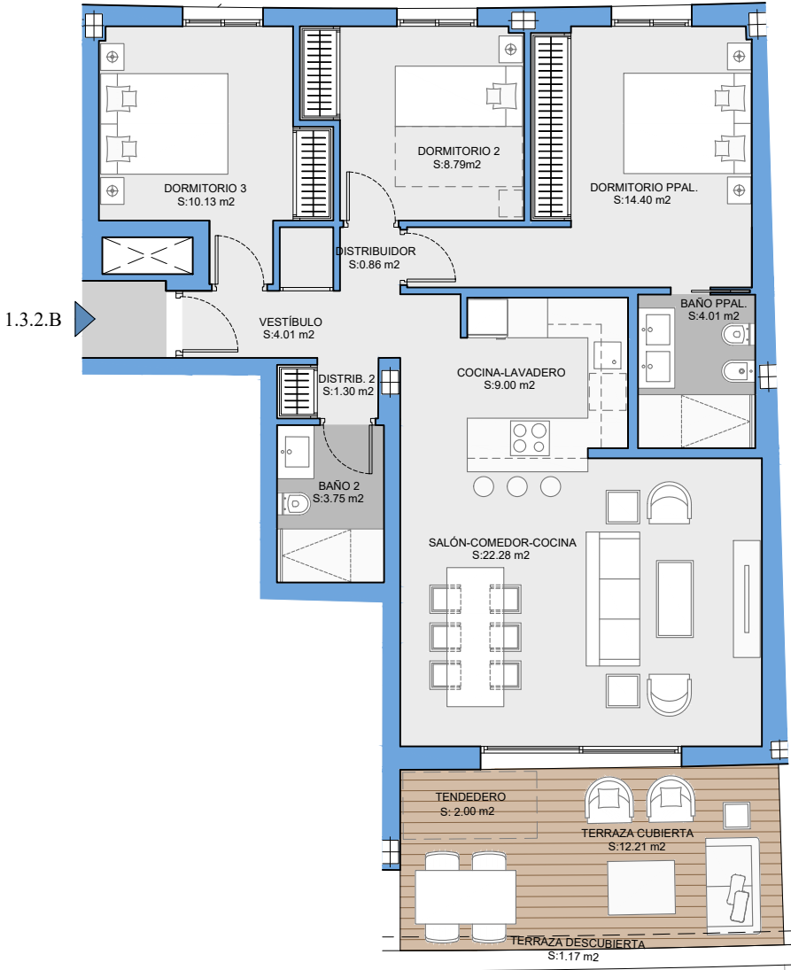
PLANTA PRIMERA
